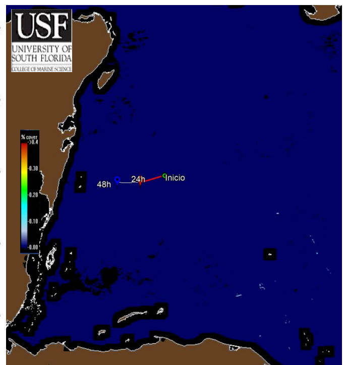
Figura 2.- Detección de 01 grupo de sargazo en la Región del Caribe Mexicano, trayectorias más cercanas a la costa, en 24 y 48 hrs. (1.0 toneladas). Densidad de algas flotantes (FAD) Universidad del Sur de Florida (USF). 20 de noviembre de 2025.
