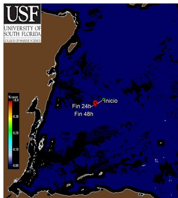
Figura 2.- Detección de 01 grupo de sargazo en la Región del Caribe Mexicano, trayectorias más cercanas a la costa, en 24 y 48 hrs. (50 toneladas). Densidad de algas flotantes (FAD) Universidad del Sur de Florida (USF). 17 de noviembre de 2025.
