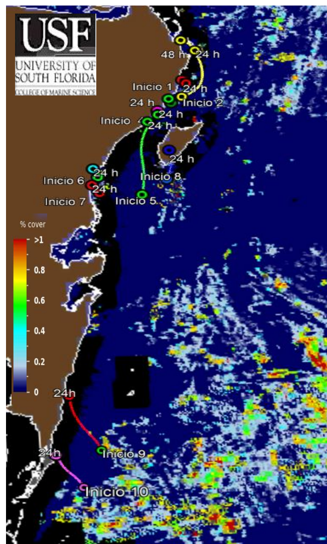
Figura 2.- 10 grupos de sargazo más cercanos a la costa de Quintana Roo (Universidad del Sur de Florida) 27 de julio de 2026. Biomasa total en el Caribe Mexicano de 38,309 Toneladas.
