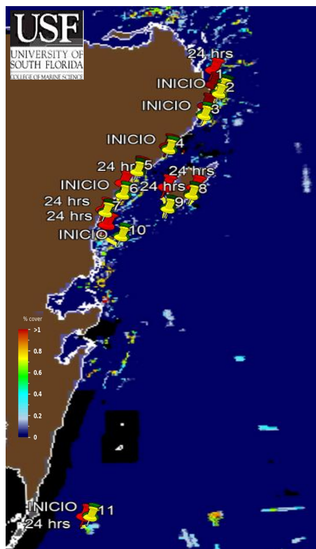
Figura 2.- 11 grupos de sargazo más cercanos a la costa de Quintana Roo (Universidad del Sur de Florida) 18 de julio de 2026. Biomasa total en el Caribe Mexicano de 25,189 Toneladas.
