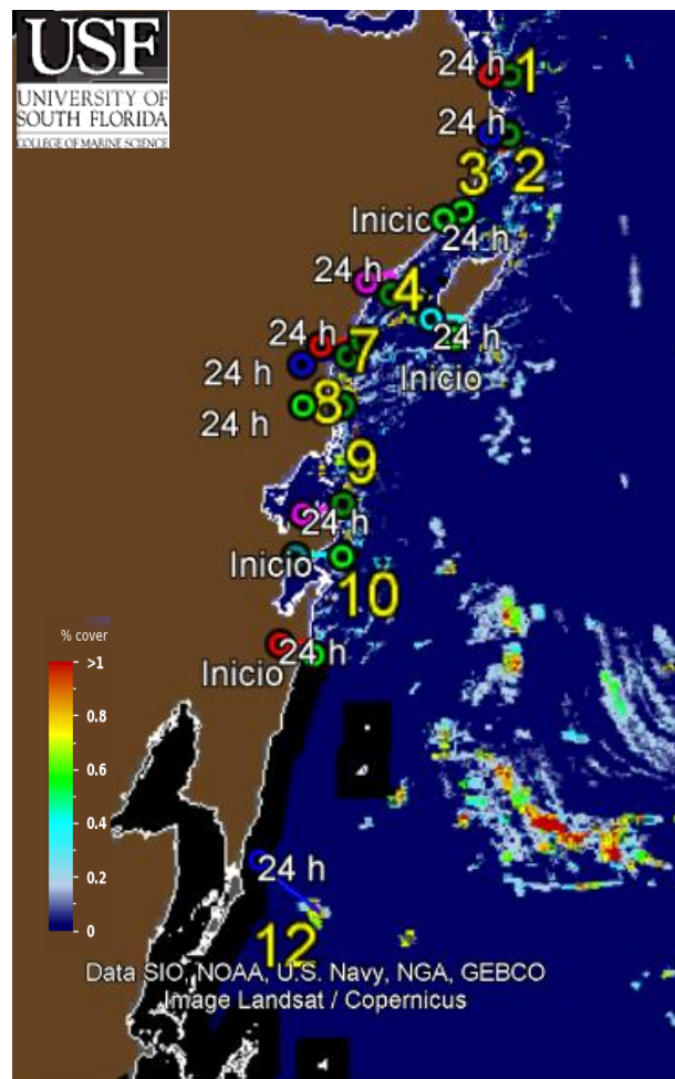
Figura 2.- 12 grupos de sargazo más cercanos a la costa de Quintana Roo (Universidad del Sur de Florida) 15 de julio de 2026. Biomasa total en el Caribe Mexicano de 13,132 Toneladas.
