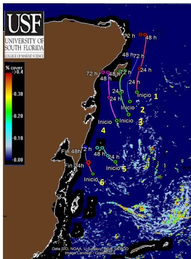
Figura 2.- 06 grupos de sargazo más cercanos a las costas de Quintana Roo (Universidad del Sur de Florida) 16 de febrero de 2026. Biomasa total en el Caribe Mexicano de 15,579 Ton.
