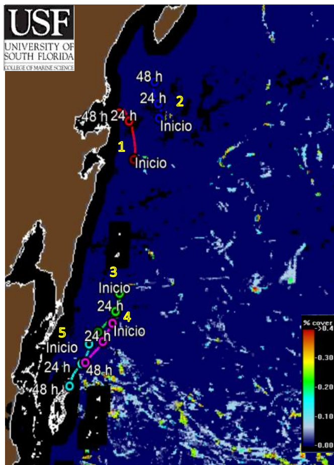
Figura 2.- 08 grupos de sargazo más cercanos a las costas de Quintana Roo. Biomasa total en el Caribe Mexicano de 12,885 Toneladas. Imágenes (Universidad del Sur de Florida) 26 de enero de 2026.
