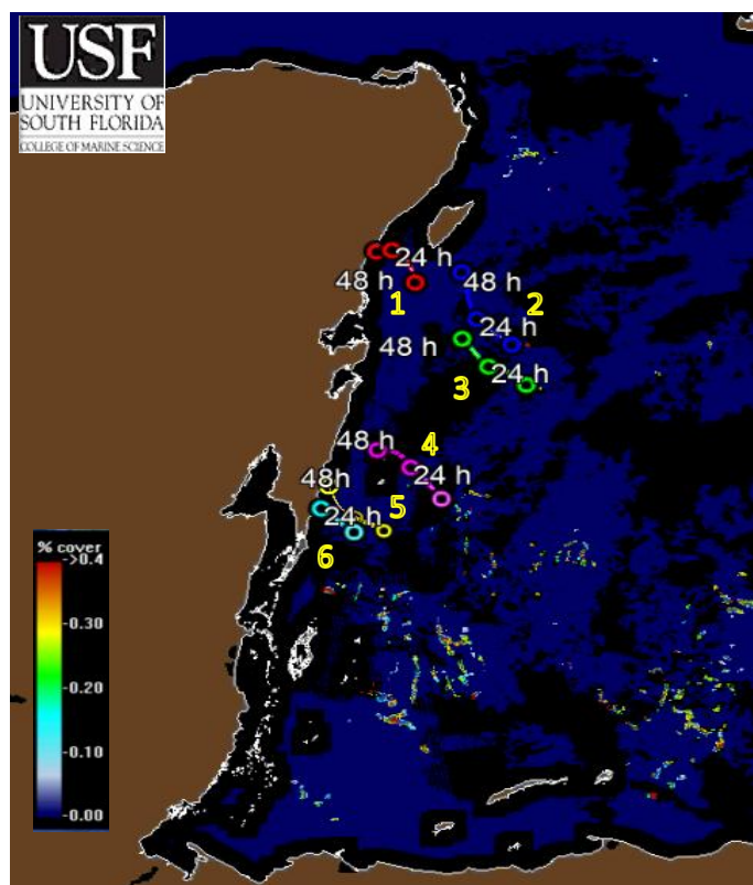
Figura 2.- 06 grupos de sargazo más cercanos a las costas de Quintana Roo. Biomasa total en el Caribe Mexicano de 3,671 Toneladas. Imágenes (Universidad del Sur de Florida) 21 de enero de 2026.
