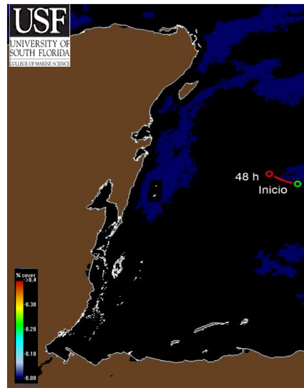
Figura 2.- 01 grupo de sargazo detectado en el Caribe Mexicano, sin posibilidad de acercarse en las próximas 24 o 48 horas a las costas de Quintana Roo. Biomasa total de 73 Toneladas, debido a la presencia de nubosidad. Imágenes (Universidad del Sur de Florida) 25 de diciembre de 2025.
