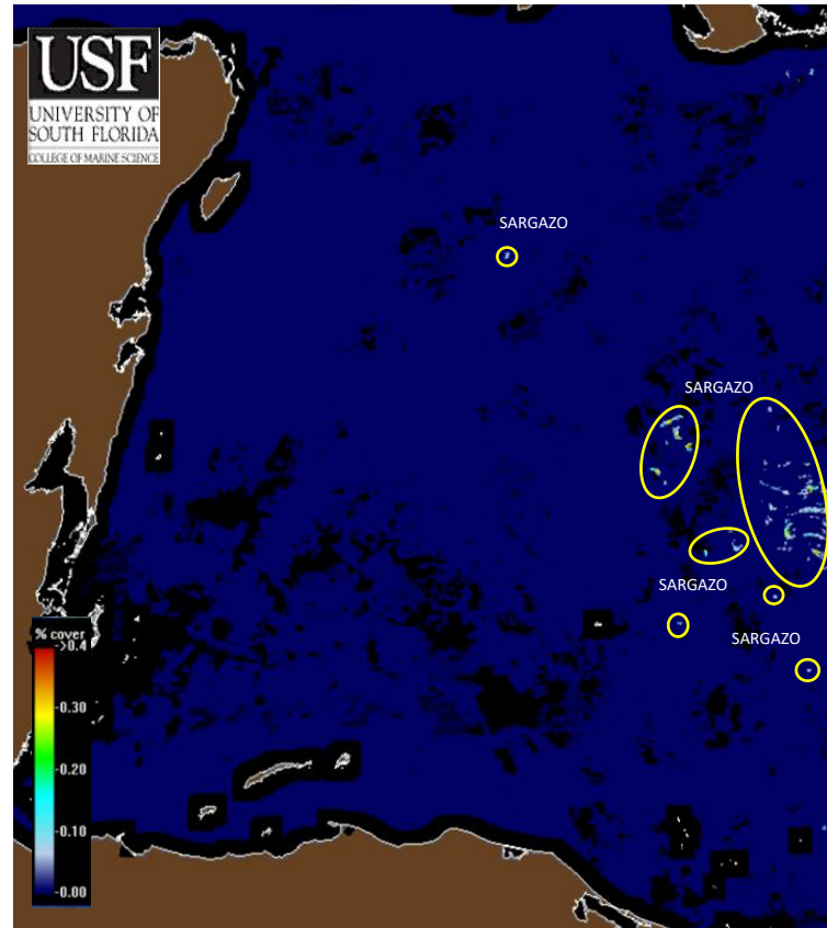
Figura 2.- Grupos detectados en el Caribe Mexicano, sin posibilidad de acercarse en las próximas 24 o 48 horas a las costas de Quintana Roo. Biomasa total de 376 Toneladas. Imágenes (Universidad del Sur de Florida) 20 de diciembre de 2025.
