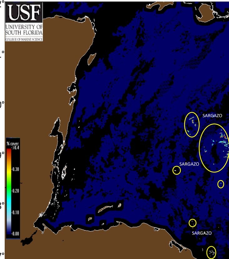
Figura 2.- Grupos detectados en el Caribe Mexicano, sin posibilidad de acercarse en las próximas 24 o 48 horas a las costas de Quintana Roo. Biomasa total de 390 Toneladas. Imágenes (Universidad del Sur de Florida) 19 de diciembre de 2025.
